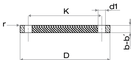
Flange Ciego
