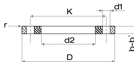
Flange Volante
